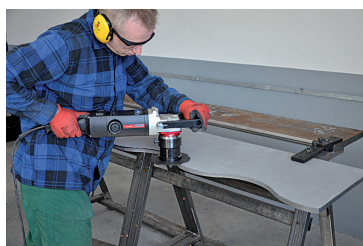
Ukosovanie hrán zakrivených tvarov
